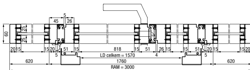
Vodorovný řez dvoukřídlymi ocelovými loftovými dveřmi s bočními díly a horním světlíkem
